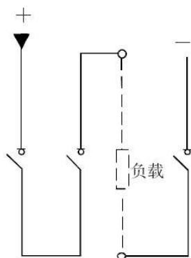
3P外形接线图(DC500V)
