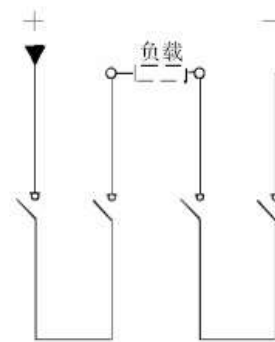
4P外形接线图(DC750V)
